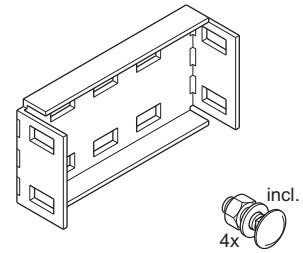
Eindschot End plate
