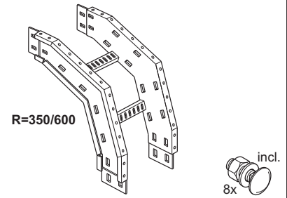
Vervalstuk 90° Vertical outer bend 90°
